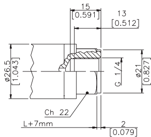
(4) G 1/4 FEMELLE
