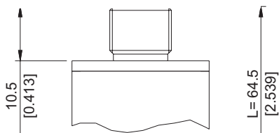
Z - Connecteur 4 pôles mâle M12 x 1
